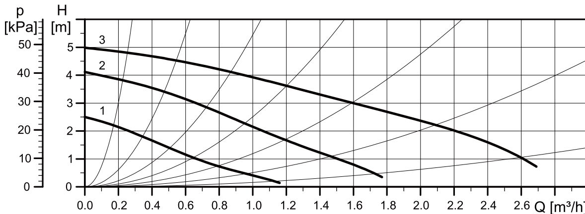
turboFLEX VUW 18-22
